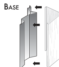
Poteau extérieur deux pièces pour les coins
